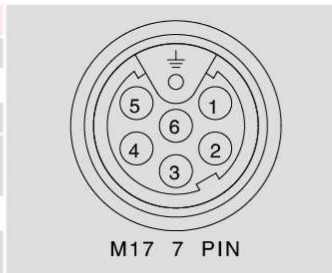
电动机动力线配国产航插 M系列接线定义
