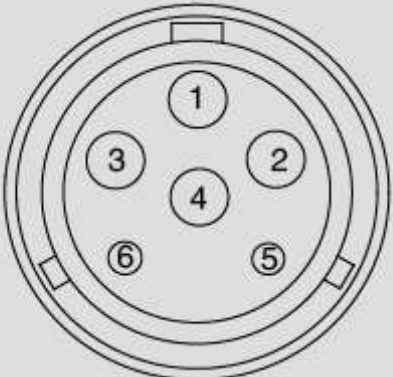
6 PIN 国产航插
