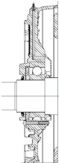
机座号 160 - 280 Motor sizes 160 - 280
