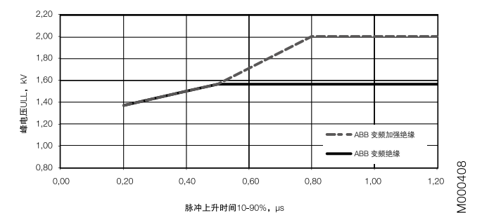
图 1 受脉冲上升时间的影响，电机端子处允许的最大相对地电压峰值
